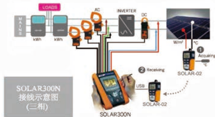
交流三相系统效率测试
