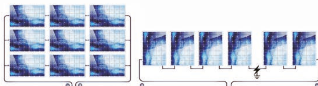
绝缘电阻测试 DUAL模式, 光伏电站接线图
