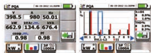
功率测量
